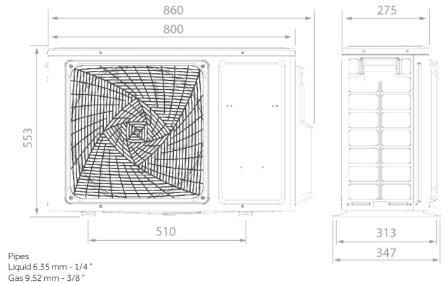
4U75S2SR5FA - 4U85S2SR5FA (4 couplings)
