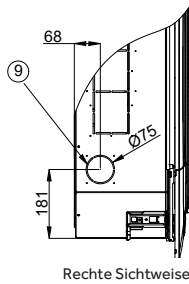
Rechte Sichtweise
