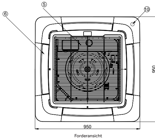
Forderansicht
