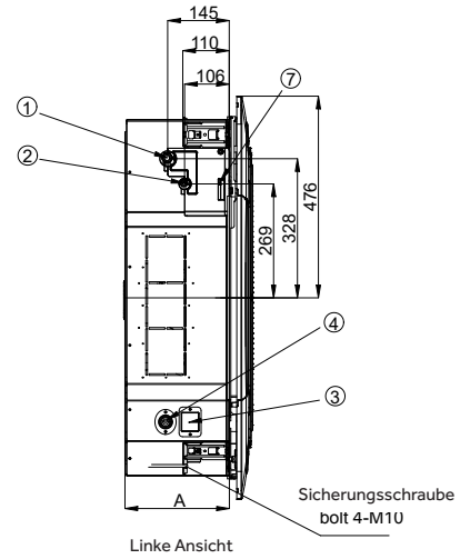
Linke Ansicht
