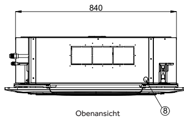
Obenansicht
